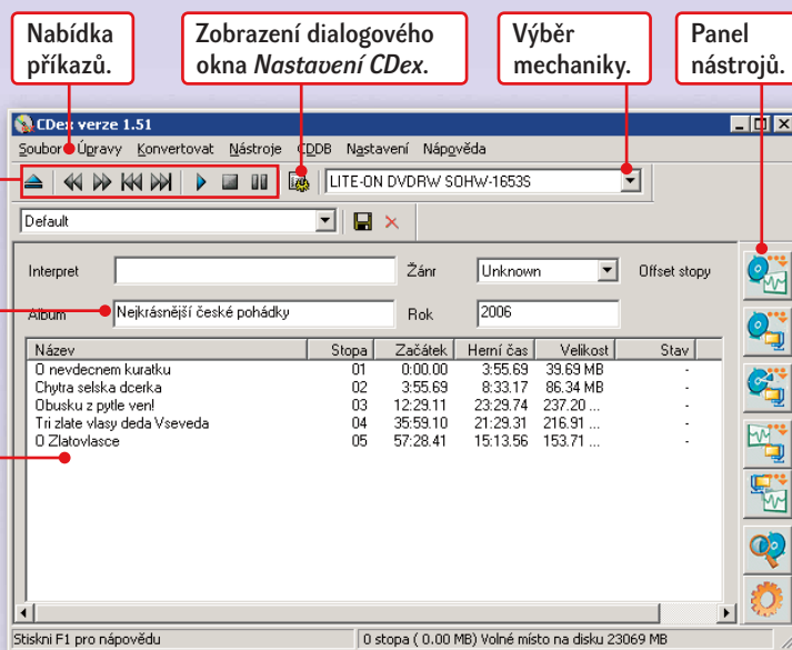
► Obr. 4. Hlavní okno programu CDex.
