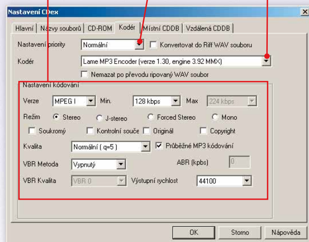
▲ Obr. 2. Dialogové okno Nastavení CDex – karta Kodér .
