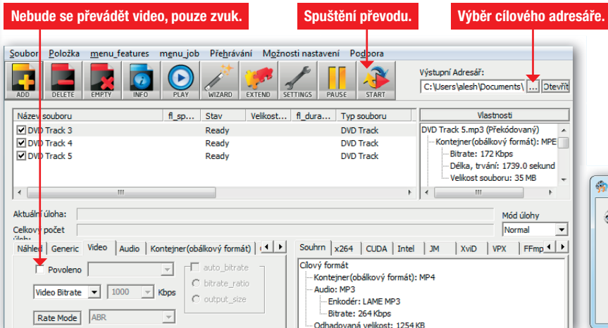
OBR. 6 Nastavení převodu.
